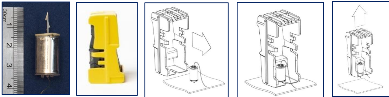
Taser Probe X10
